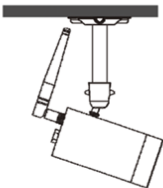
Deckenmontage
